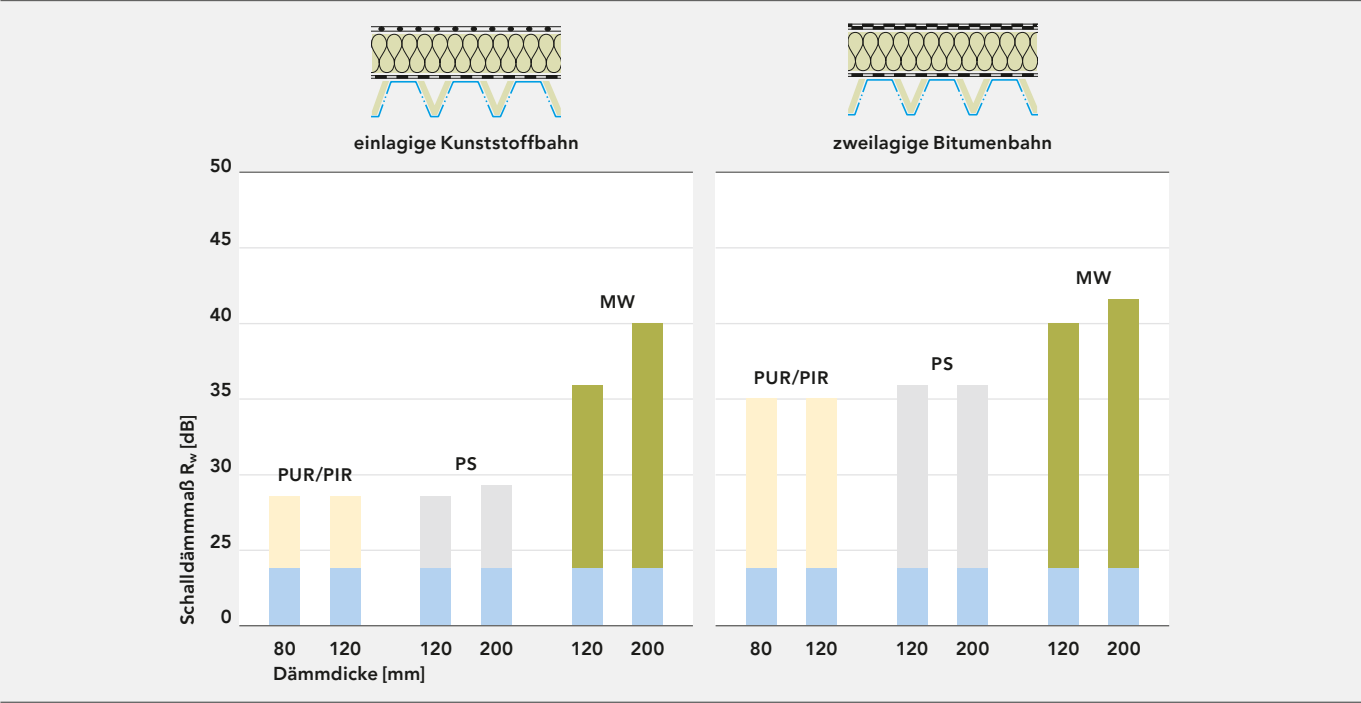
Schalldämmmaß bei Akustik-Trapezprofilen (gelocht)
