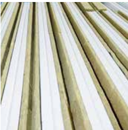
Einlegen von Akustik-Profilfüllern in Trapezprofile
