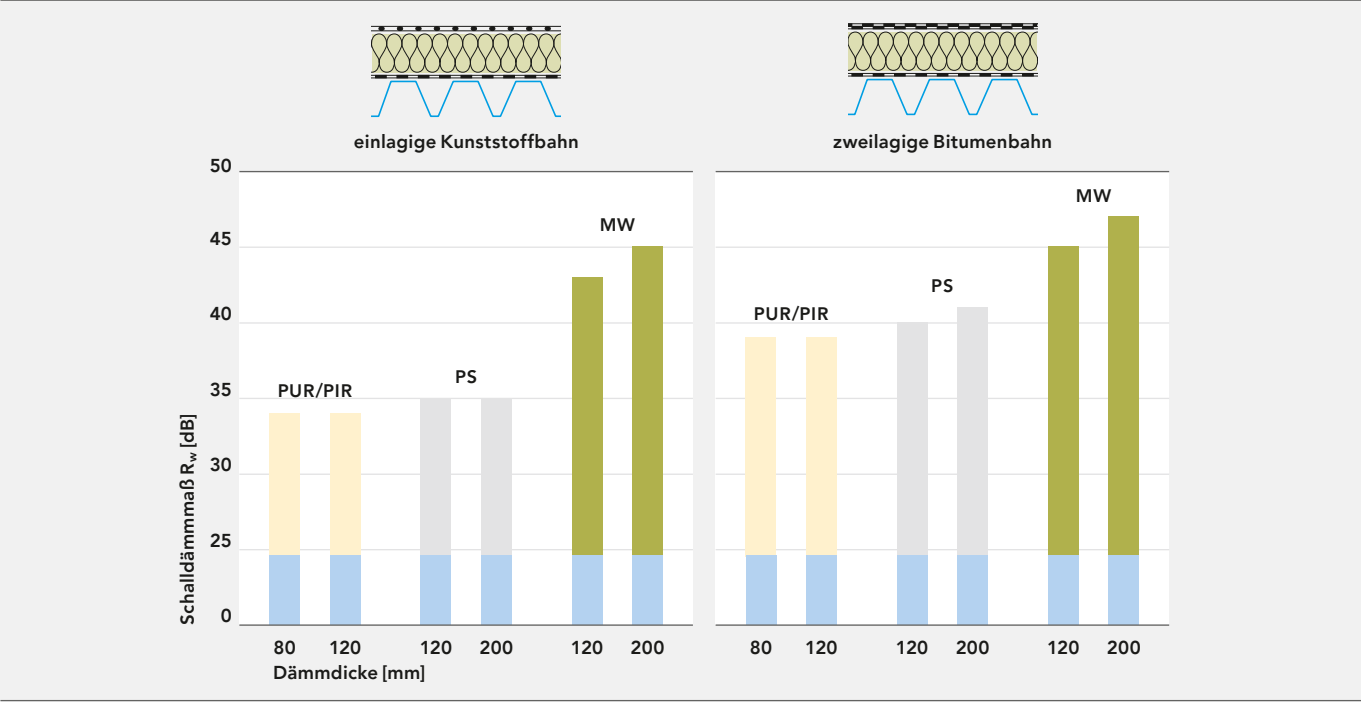
Schalldämmmaß bei Trapezprofilen (ungelocht)
